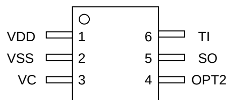
TTP118-CA6 SOT23-6
